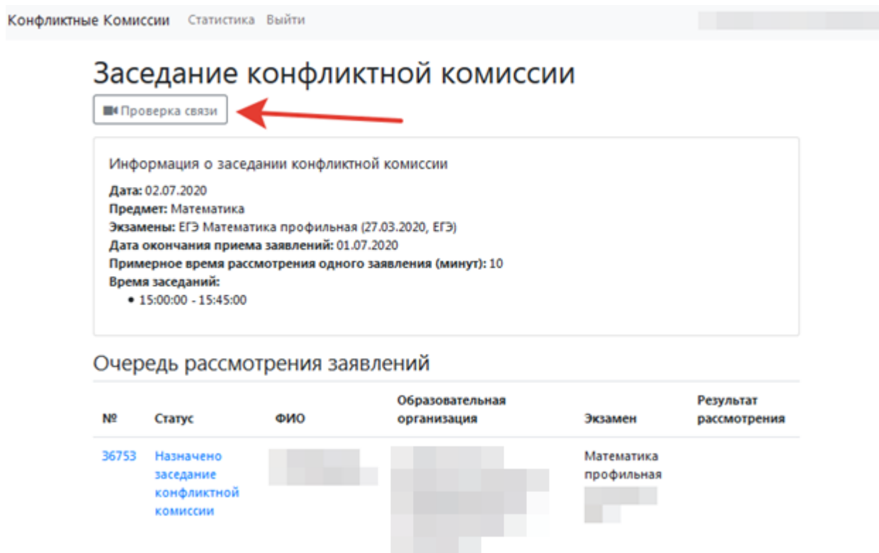
Рисунок 8 – Проверка связи
