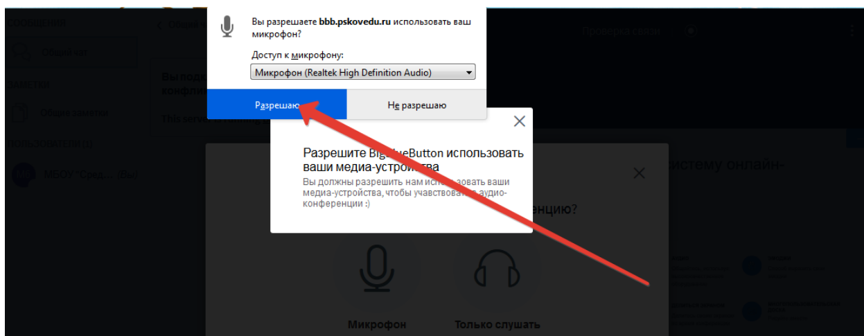
Рисунок 11 – Использование медиа-устройств
